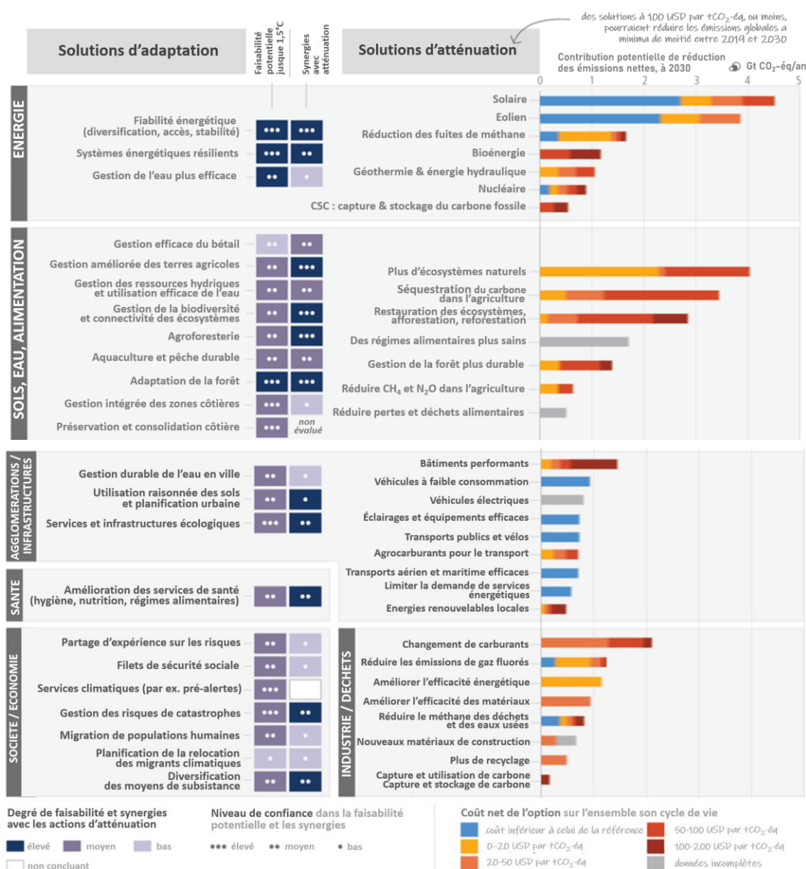
Figure 6. Faisabilité des réponses au changement climatique et des options d'adaptation, et potentiel d'options d'atténuation à court terme.
